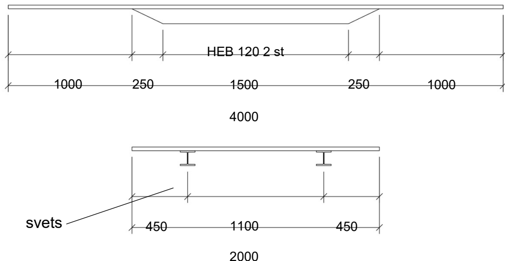
Figur 52-5 Förstärkning med två I-balkar
