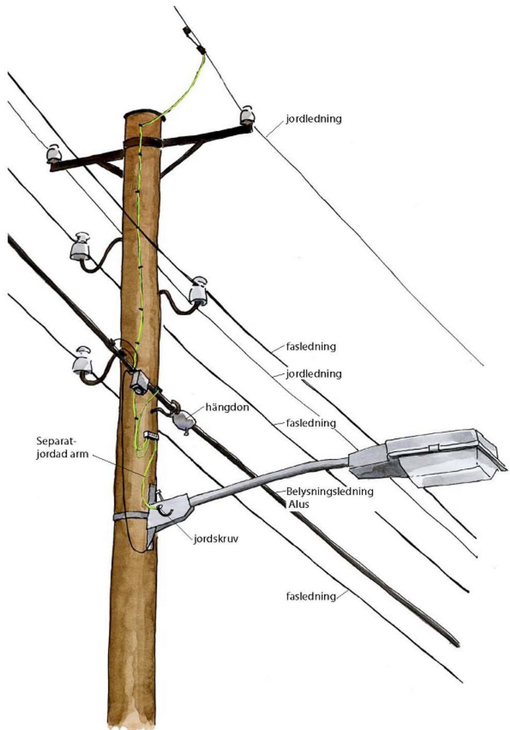
Figur 42-9 Friledning el & alus belysning
